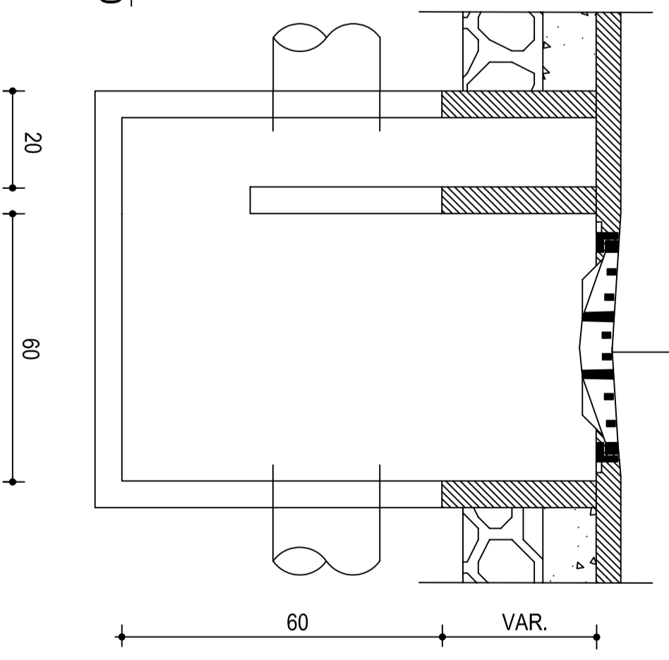
SEZIONE A-A
